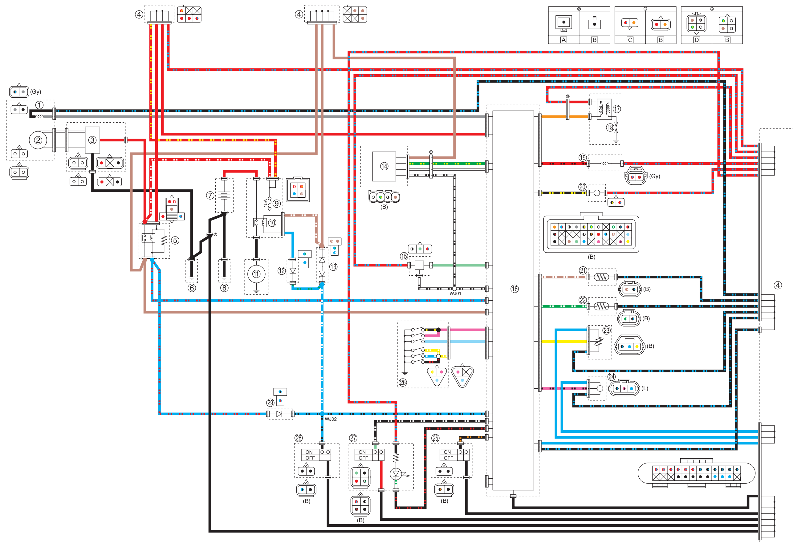
YZ250F/YZ250FP 2023 WIRING DIAGRAM
